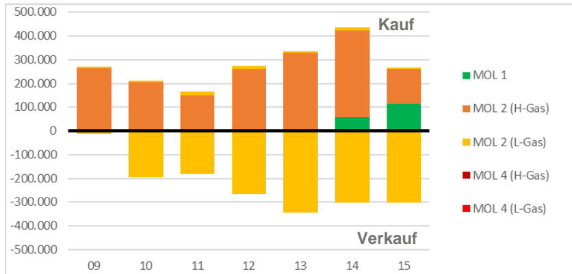
Externer Regelenergieeinsatz in KW 02 (09.01.-15.01.) in MWh/d
