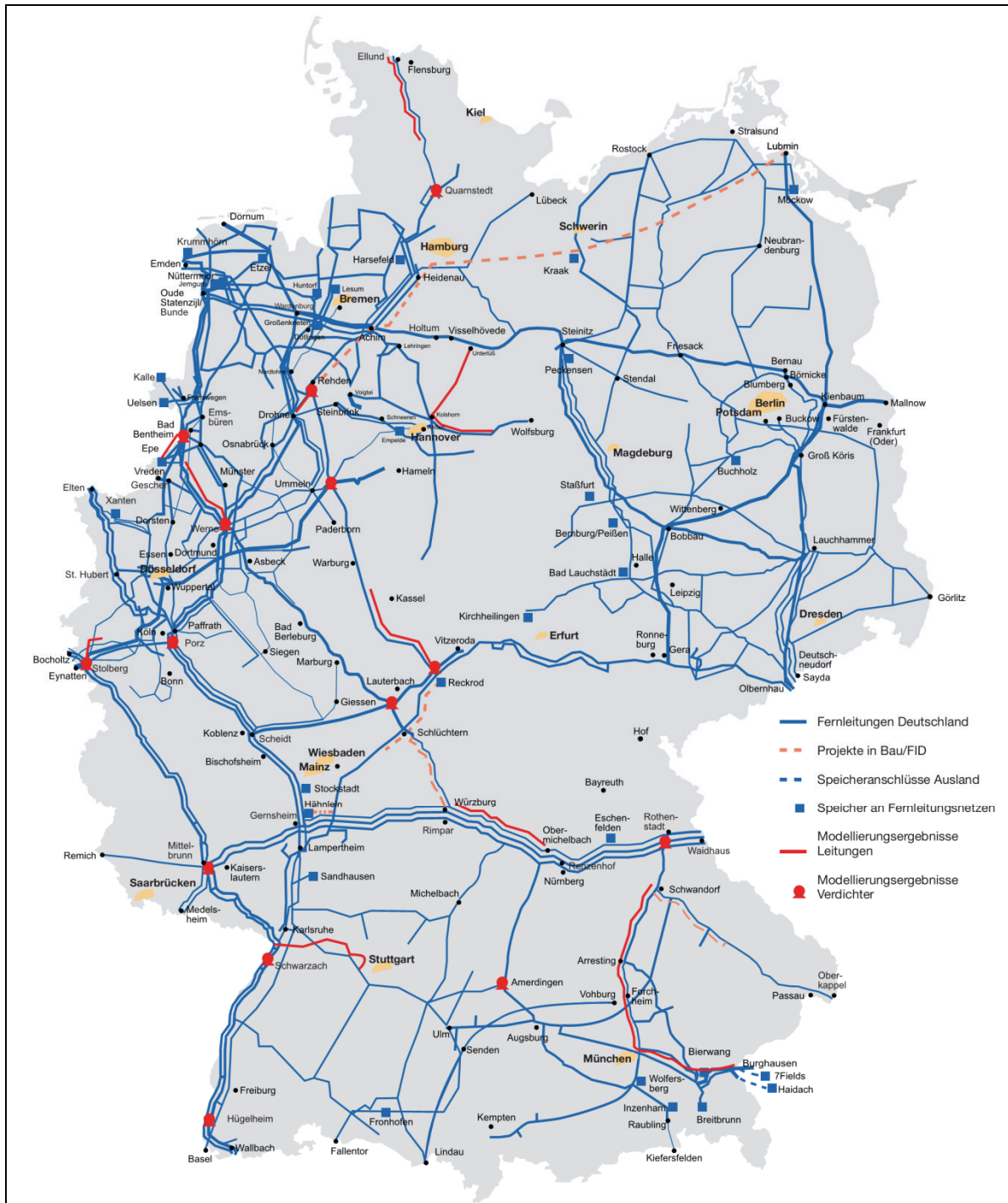
Abbildung 21: Ergebnis-Übersicht für 2022 im Szenario II
