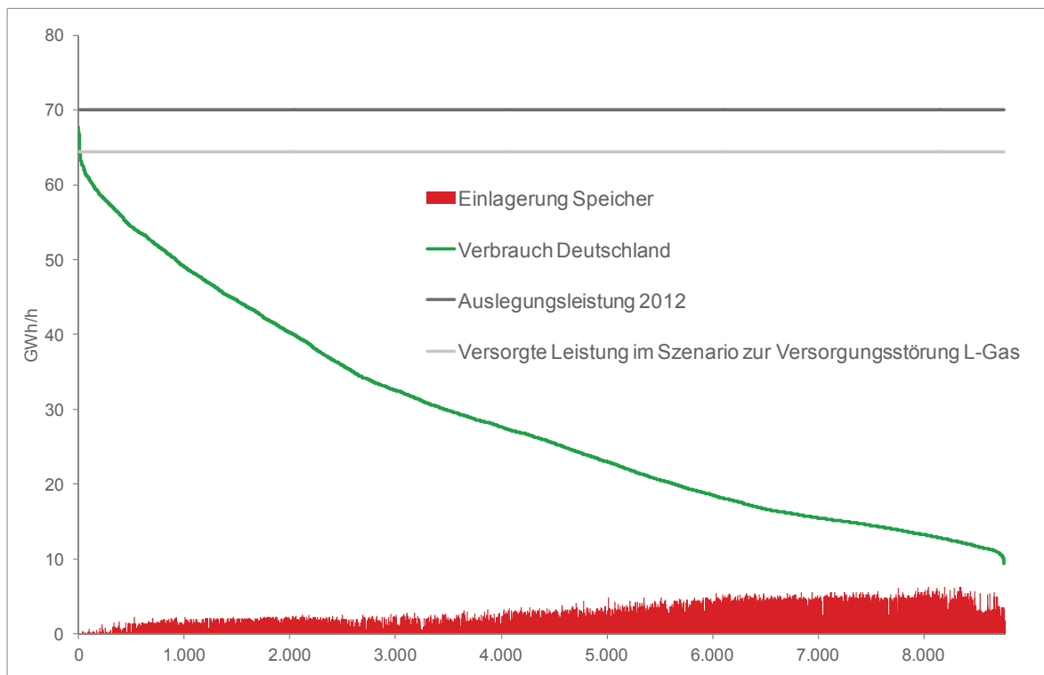
Abbildung 27: Gegenüberstellung Verbrauch L-Gas 2009/2010 in Deutschland und Auslegungsleistung des Gasnetzes
