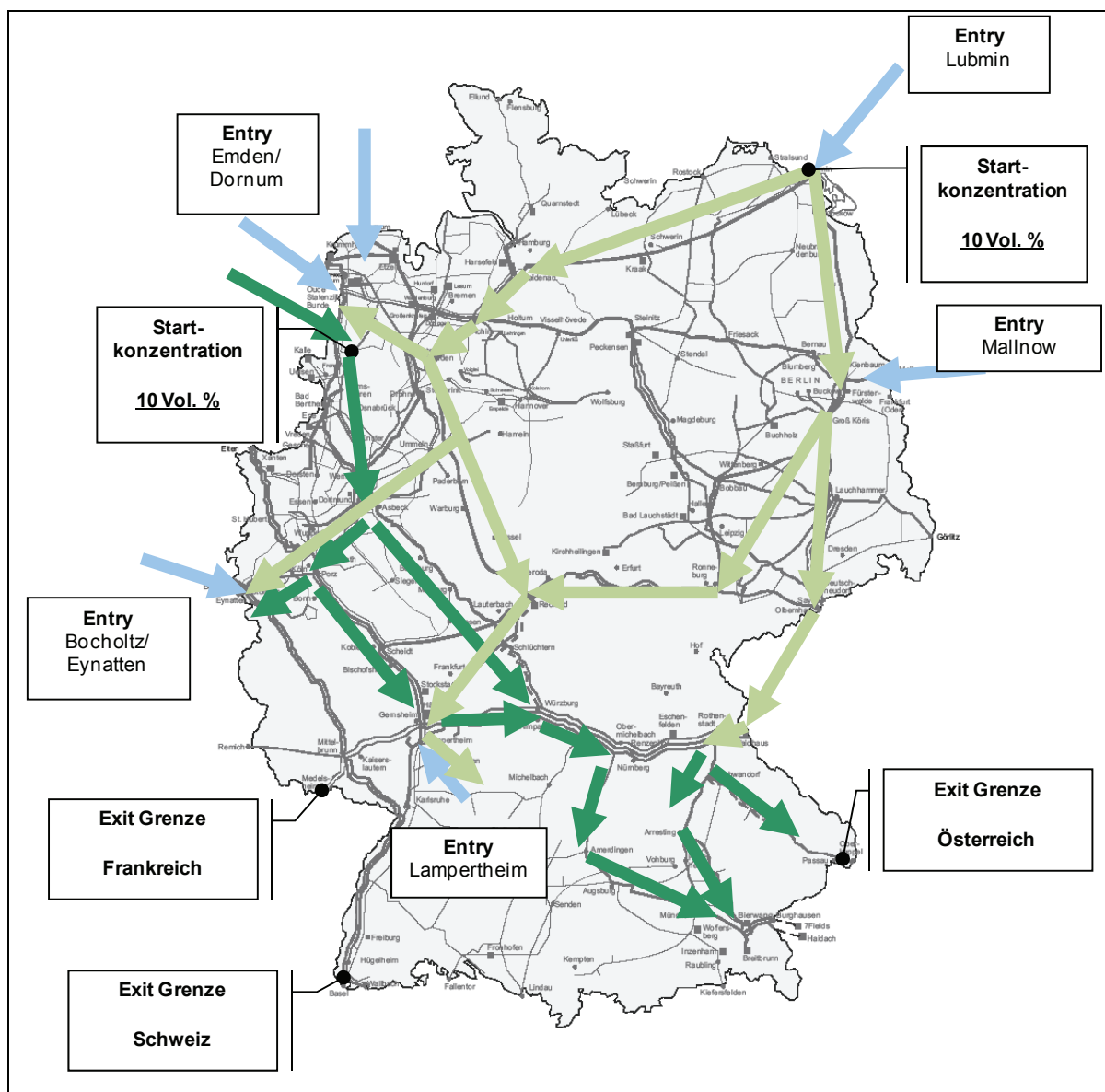
Abbildung 24: Verlauf des Wasserstoffs in Deutschland
