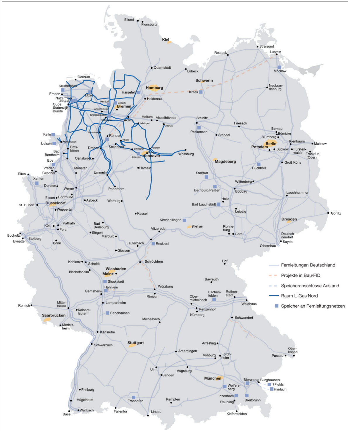
Abbildung 17: Raum L-Gas Nord (Szenario II)
